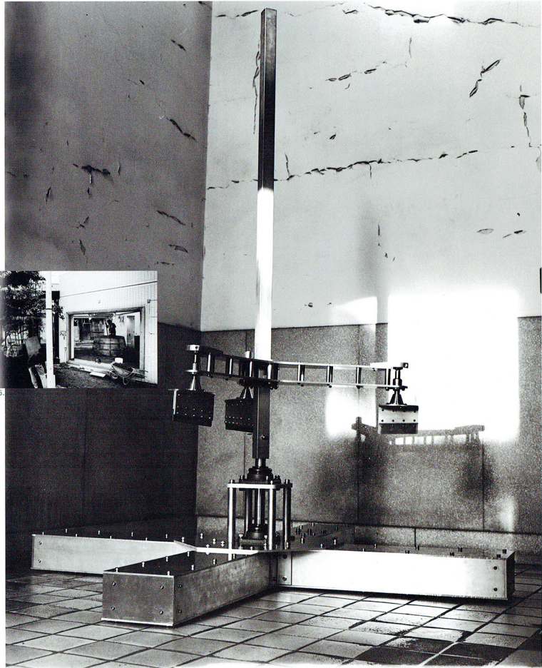
14. Homage to the Moonの動力装置部分 1991
